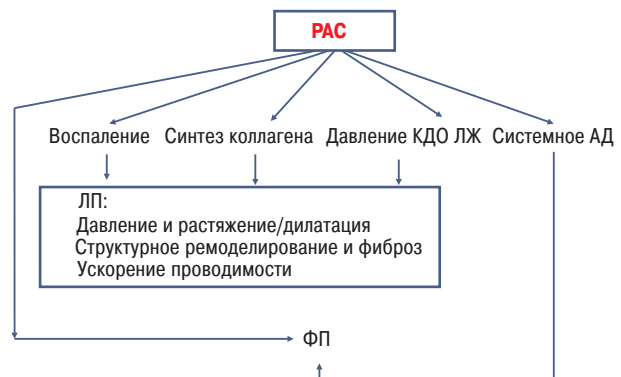
Рисунок. Механизмы влияния РАС на развитие ФП. КДО ЛЖ — конечный диастолический объем левого желудочка
